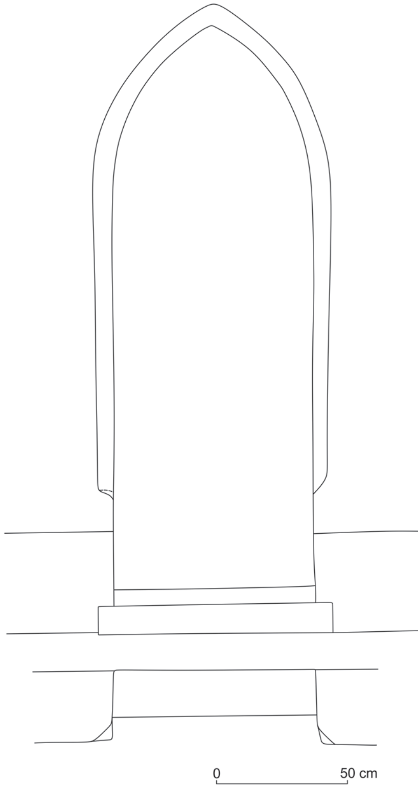
Ivaničná - pôdorys kostola
