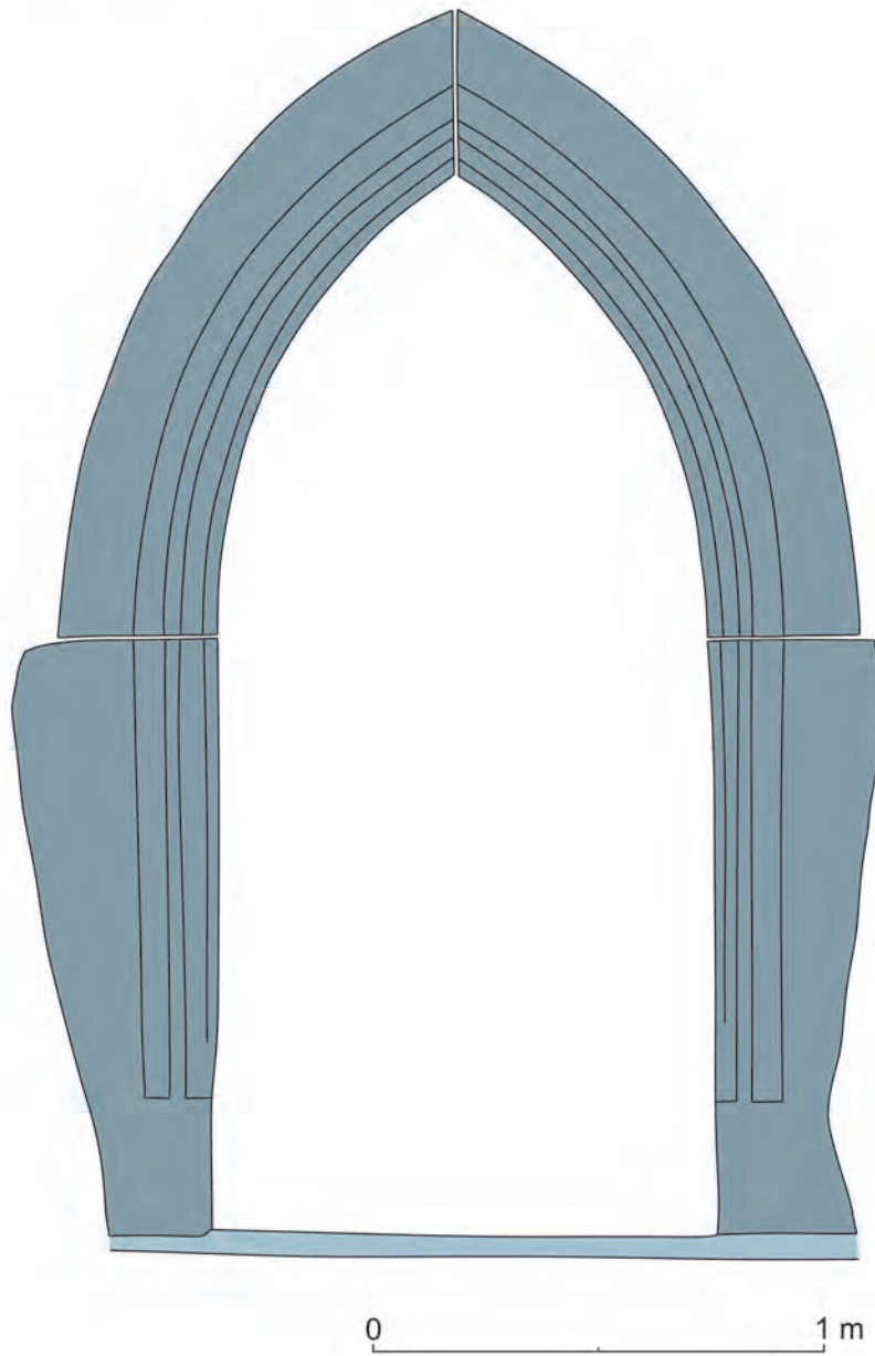
Veľká Čalomija - portál kostola
