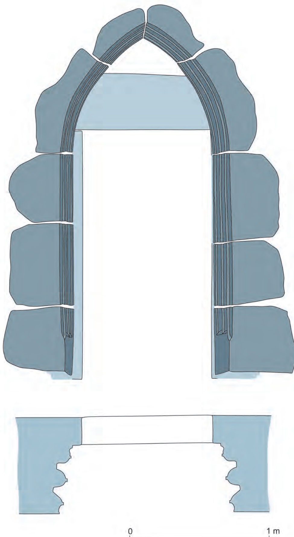
Sklabiňa - portál kostola
