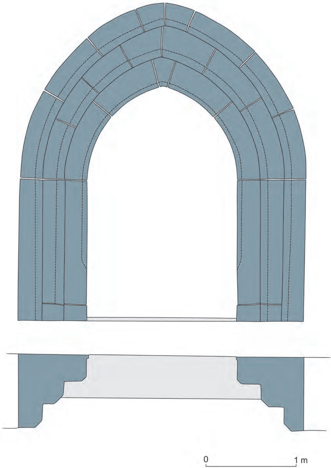
Martin -portál kostola
