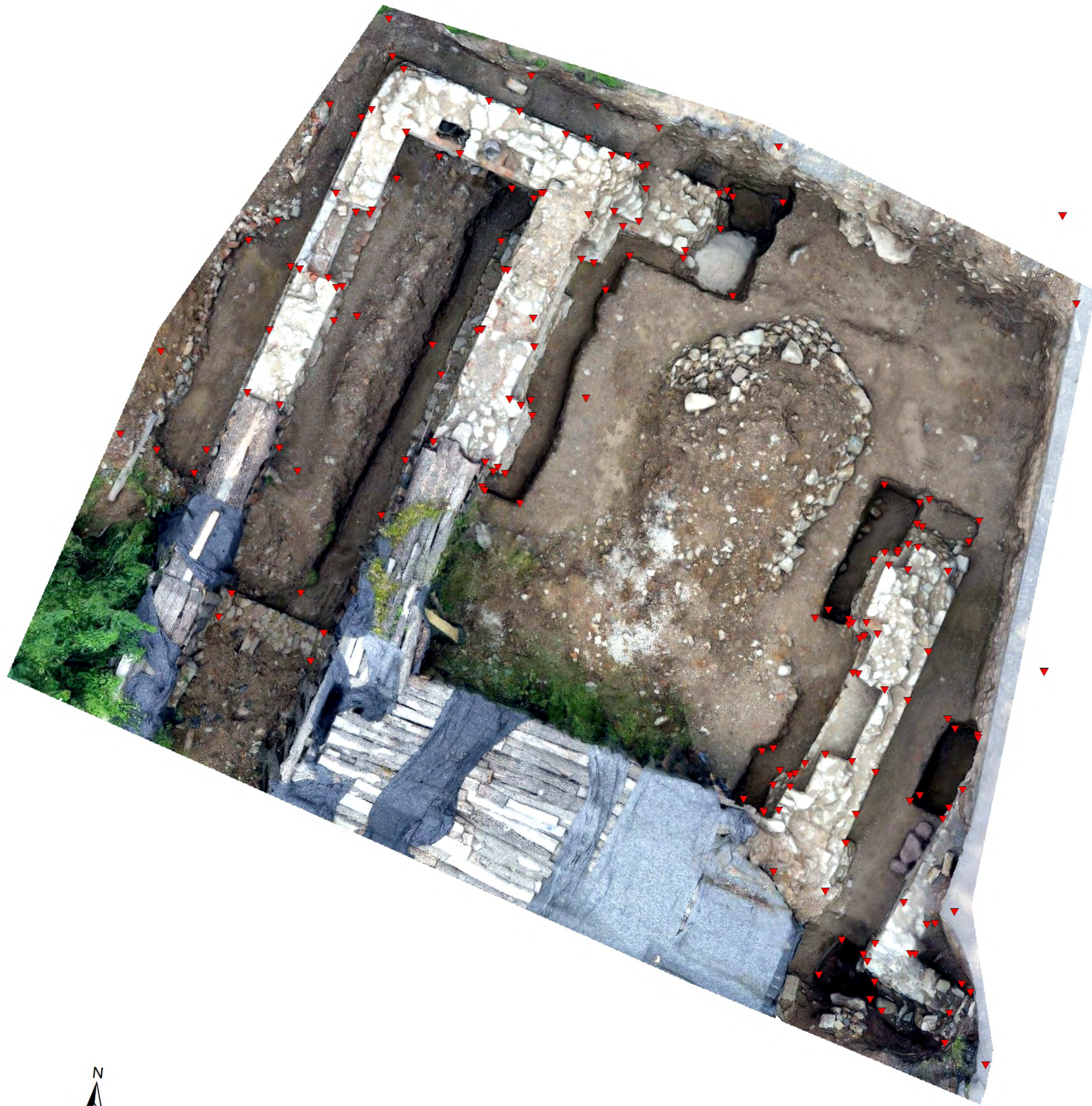
geodetické zameranie vsadené do 3D fotogrametrie
