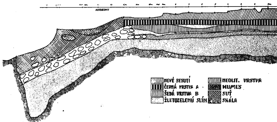
Obr. 1. Bánov. Profil se zbytky kamenné zdi. Výzkum 1943.
