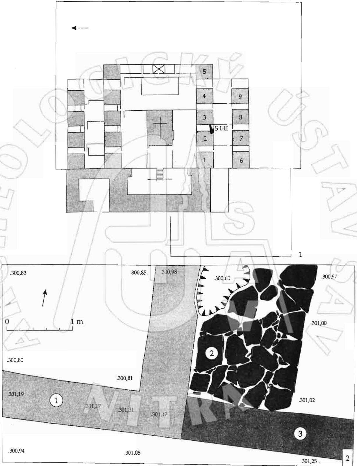
Obr. 145. Nitra-Zobor (areál bývalého Zoborského kláštora). 1 - pôdorys barokového kláštora sv. Jozefa (upravené podľa Habovštiak 1971) s vyznačením skúmanej plochy; 2 - sonda II/01. Pôdorys odkrytých murív: 1 - SV nárožie mníšskeho príbytku; 2 - exteriérová kamenná dlažba; 3 - základové múrivo ohradového múru (Samuel, 178).
