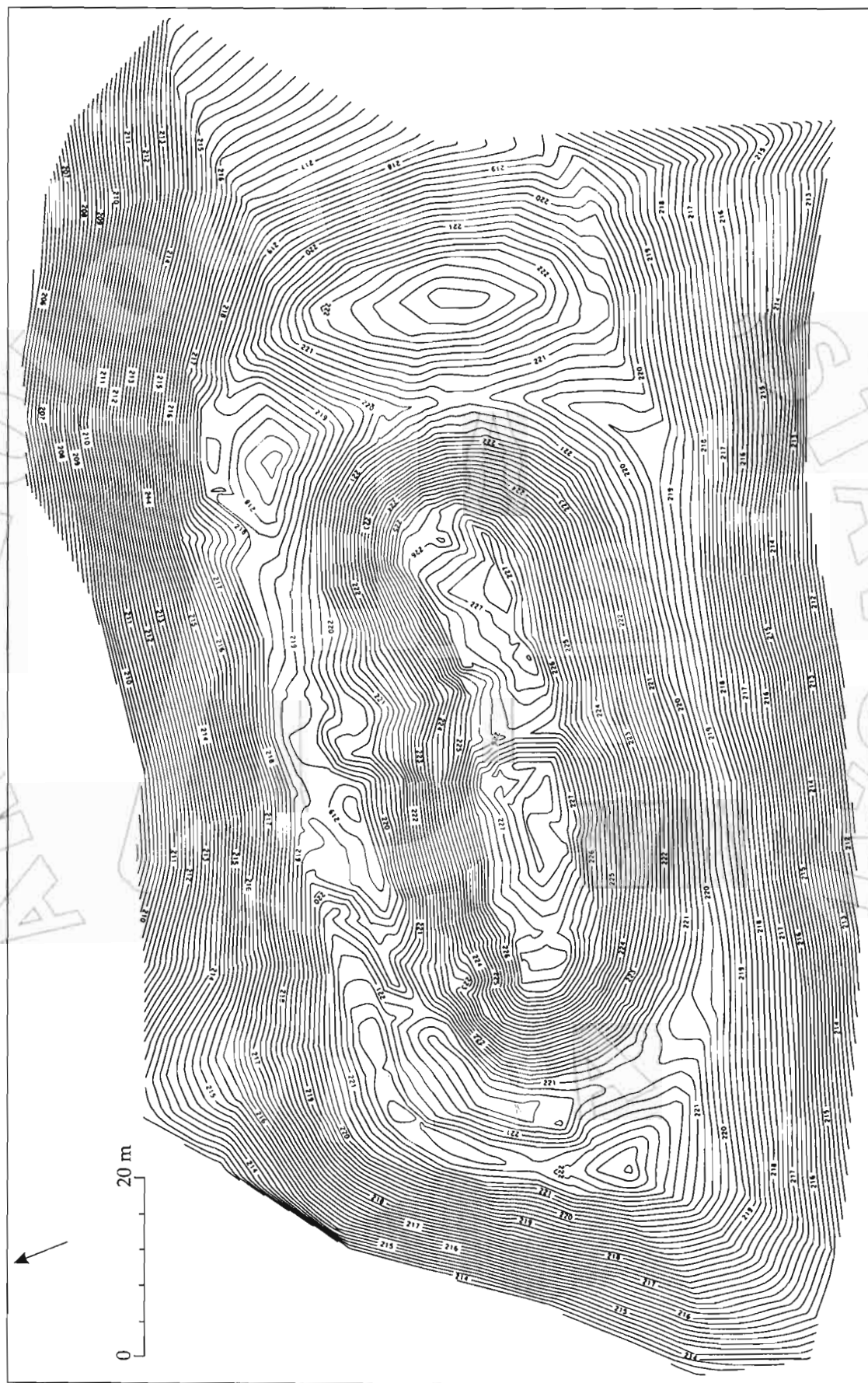
Obr. 45. Malé Zlievce (Várhegy). Tachymetrický plán lokality (Hunka/Nevizánsky/Ozdáni, 74) Abb. 45. Malé Zlievce (Várhegy). Tachymetrischer Plan der Lokalität (Hunka/Nevizánsky/Ozdáni, 74).
