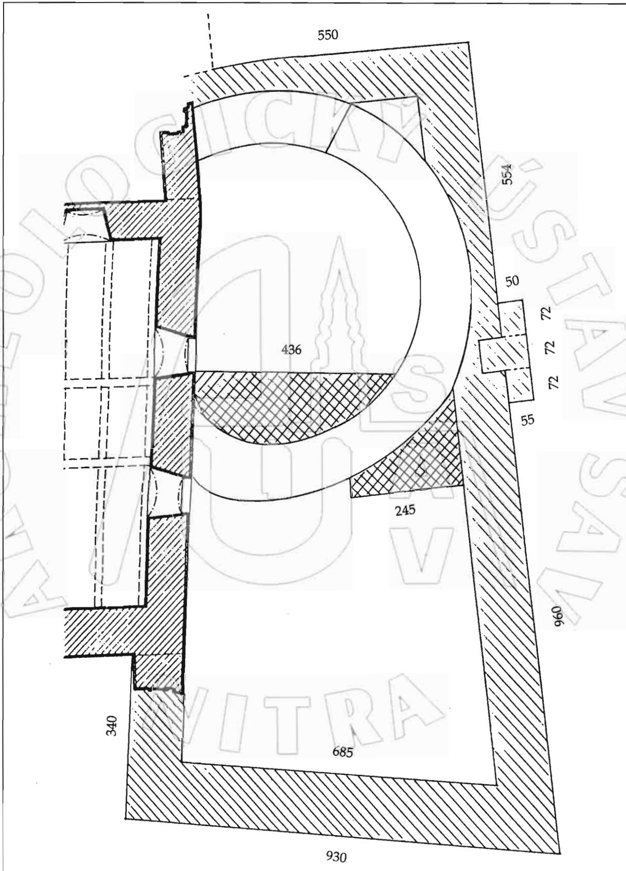
Obr. 52. Borša. Základy okrúhlej stavby a juhozápadnej nárožnej veže (Chovanec, 77). Abb. 52. Borša. Fundamente des runden Baues und des südwestlichen Eckturmes (Chovanec, 77).
