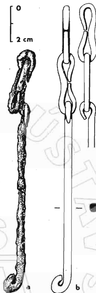
Obr. 164. Studienka. a - železná reťaz z výplne obj. 12/81; b - rekonštrukcia pôvodného vzhľadu reťaze /súčasť závesnej reťaze kotlíka?/. (L. Zachar, s. 309)
