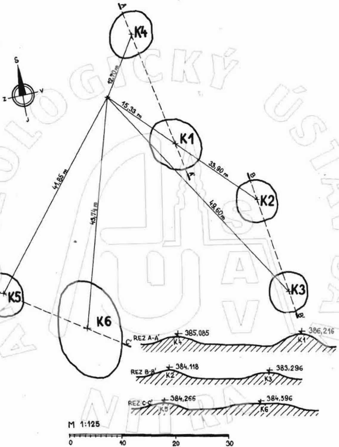
Obr. 110. Trenčín, časť Kubrá, okr. Trenčín. Rozmiestnenie, pôdorysy a rezy veľkých mohýl prvej skupiny
