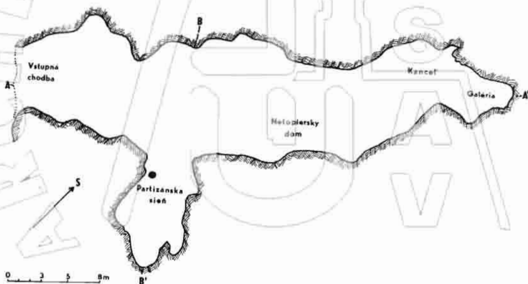
Obr. 96. Banská Bystrica, časť Sásová /Netopierska jaskyňa/. Plán jaskyne /zameraný r. 1951 a 1955 J. Bárta/. Miesto nálezu je vyznačené krúžkom
