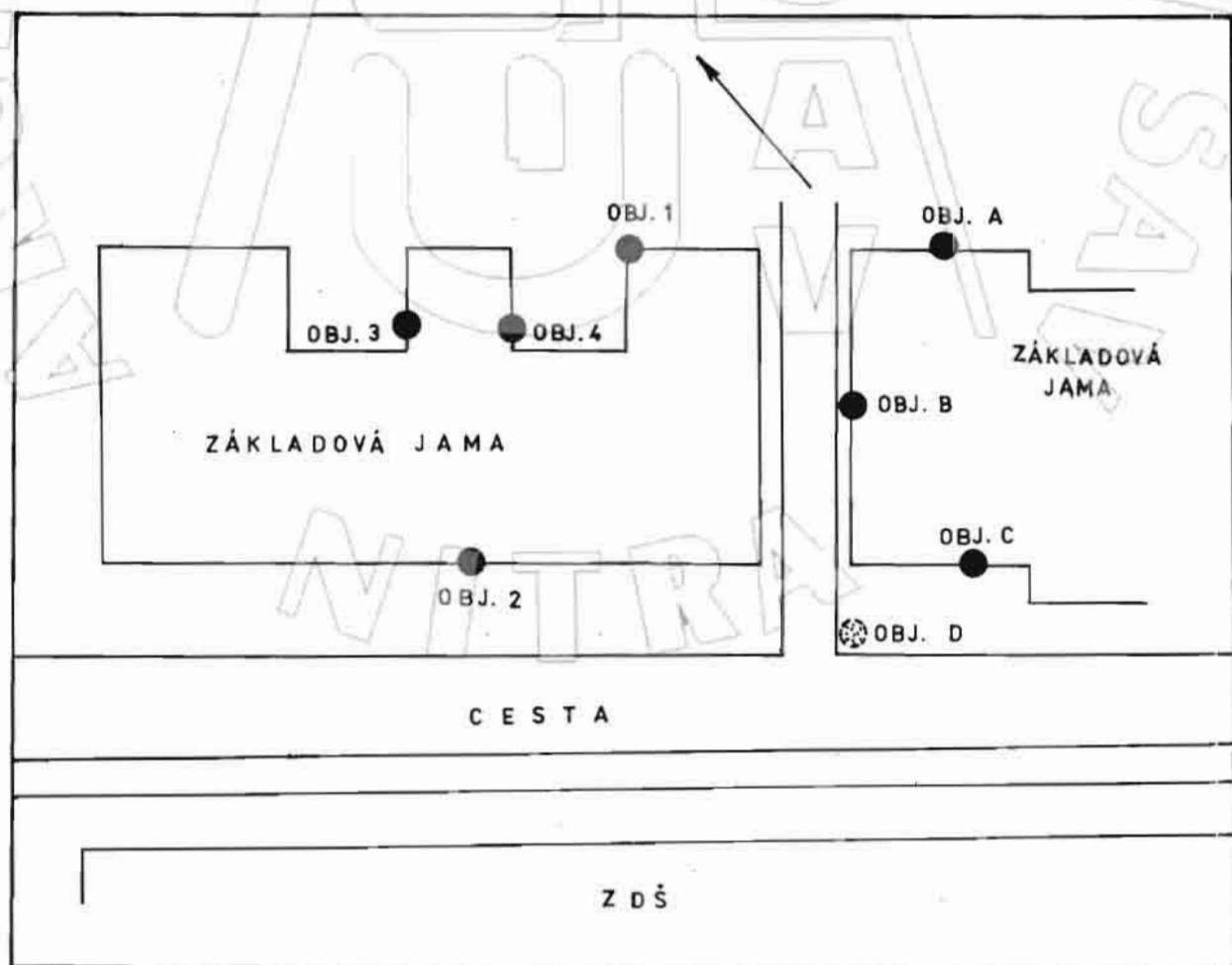
Obr. 145. Vrbové, okr. Trnava. Pôdorysný náčrt základových jám s objektmi
