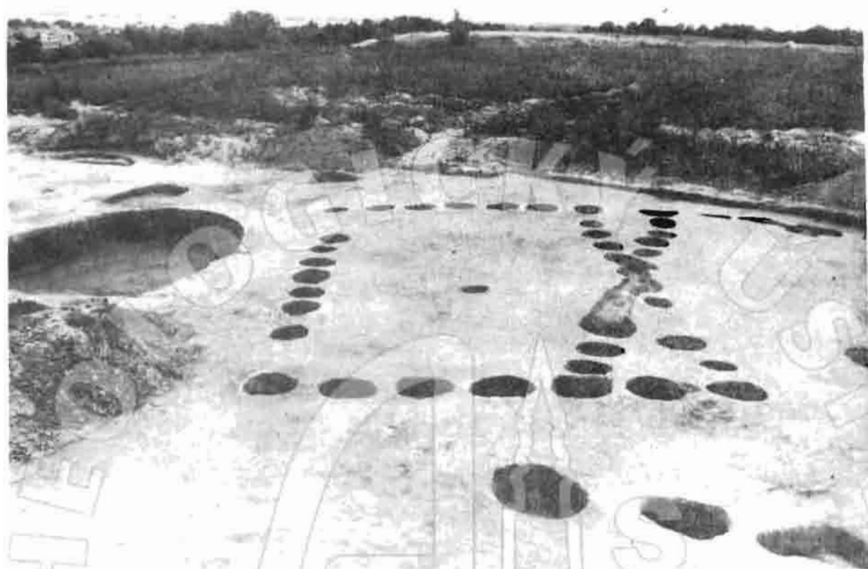
Obr. 121. Zlkovce, okr. Trnava. Severná časť kolových stavieb lengyelskej kultúry od S
