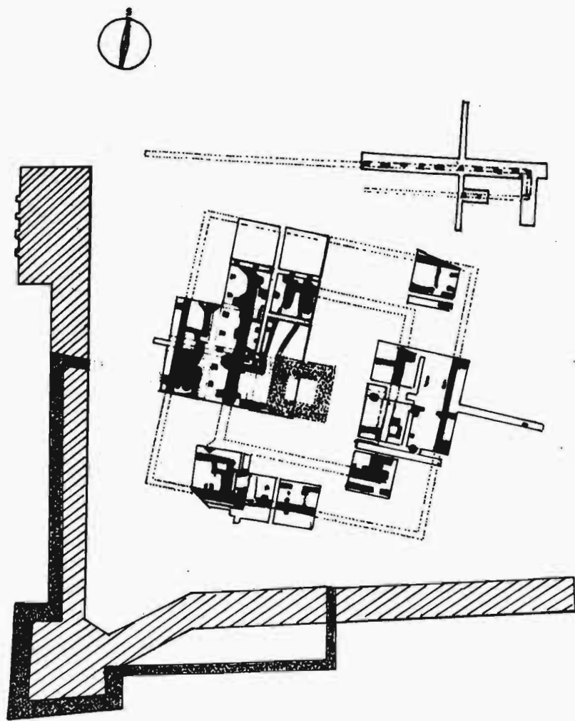
Obr. 4. Sereď. Nádvorie kaštieľa. Celkový plán archeologického výskumu do r. 1988.
