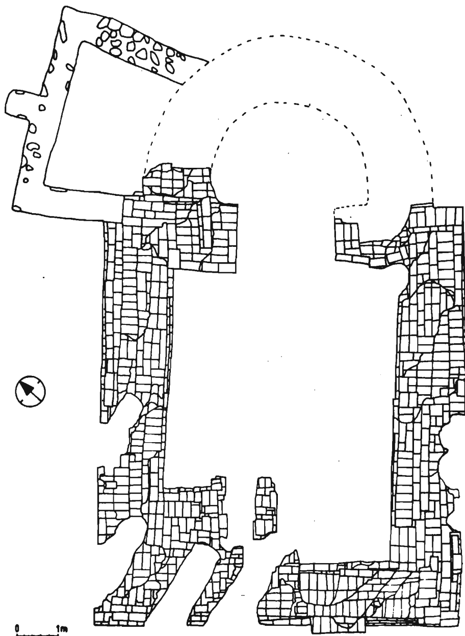
Obr. 2. Pinciná, okr. Lučenec. Základy stredovekého kostola.
